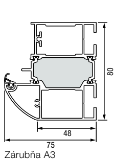
Zárubňa A3
