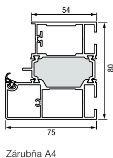
Zárubňa A4
