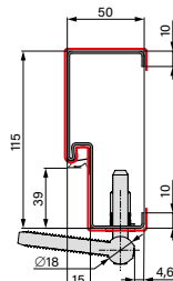
OCELOVÁ ZÁRUBŇA
