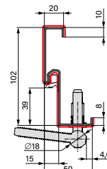
ROHOVÁ OCELOVÁ ZÁRUBŇA
