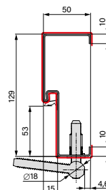
OCELOVÁ ZÁRUBŇA
