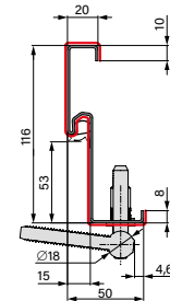
ROHOVÁ OCELOVÁ ZÁRUBŇA
